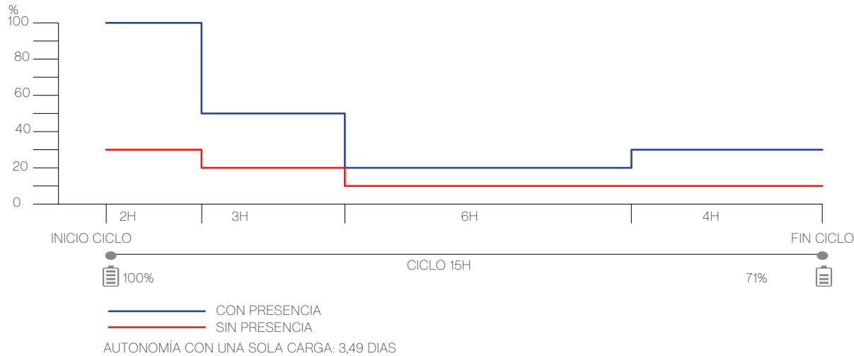
CURVA DE PROGRAMACIÓN Nº 1 (4 TRAMOS DE TIEMPO CON DETECCIÓN) PROGRAMMING CURVE #1 (4 TIME STAGES WITH DETECTION)
