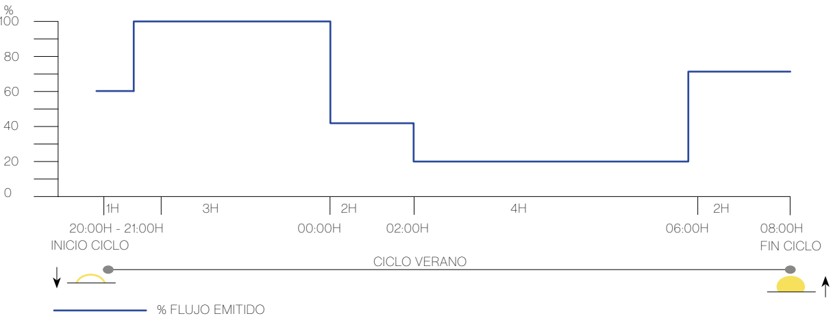
CURVA DE PROGRAMACIÓN 5 NIVELES (CILO DE VERANO)
